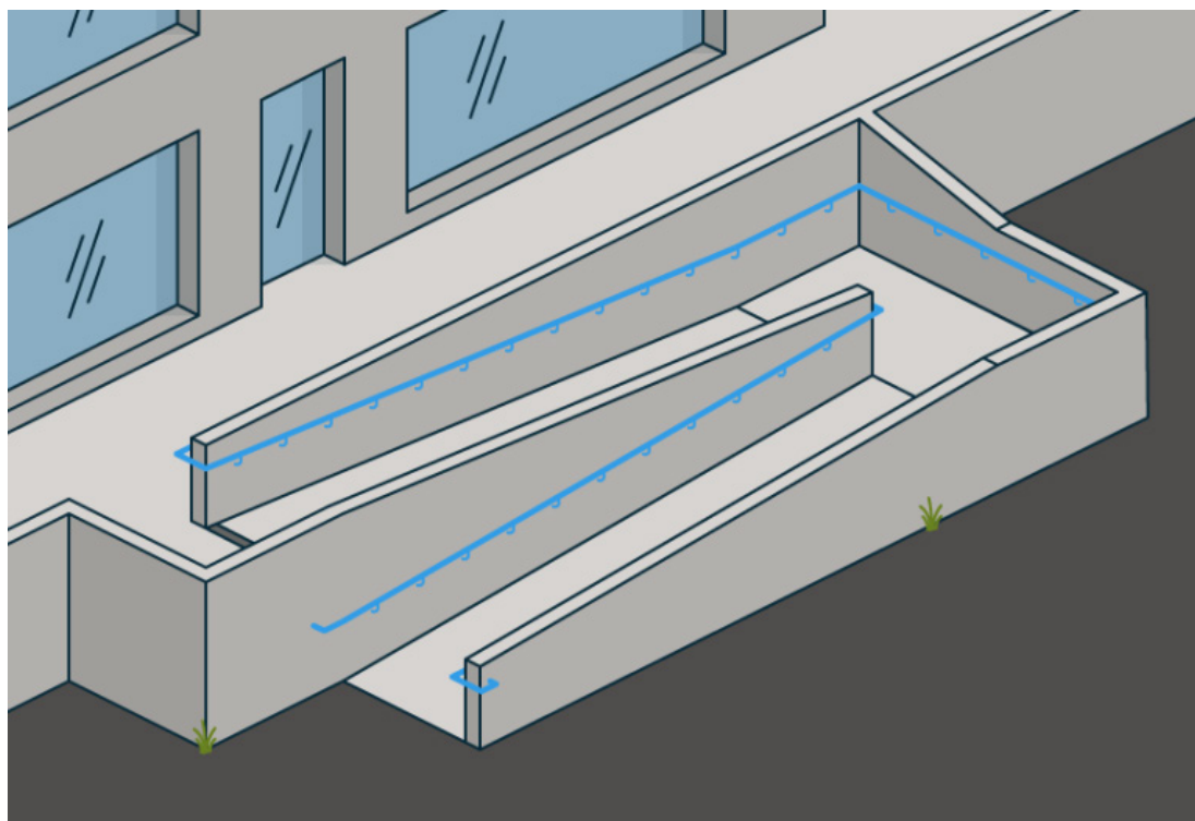
§ 12-16 Figur 2: Eksempel på rampe med håndløper i én høyde (tredje ledd) og luminanskontrast både ved toppen og bunnen av det skrå planet (fjerde ledd).
