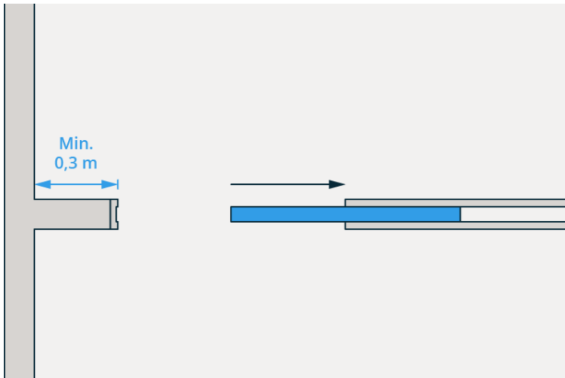
§ 12-13 Figur 5: Nødvendig fri sideplass ved skyvedør.
