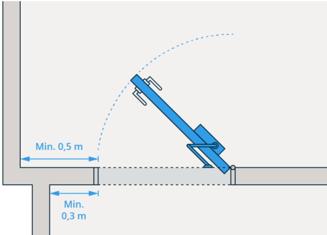
§ 12-13 Figur 6: Nødvendig fri sideplass ved dør med belastning.
